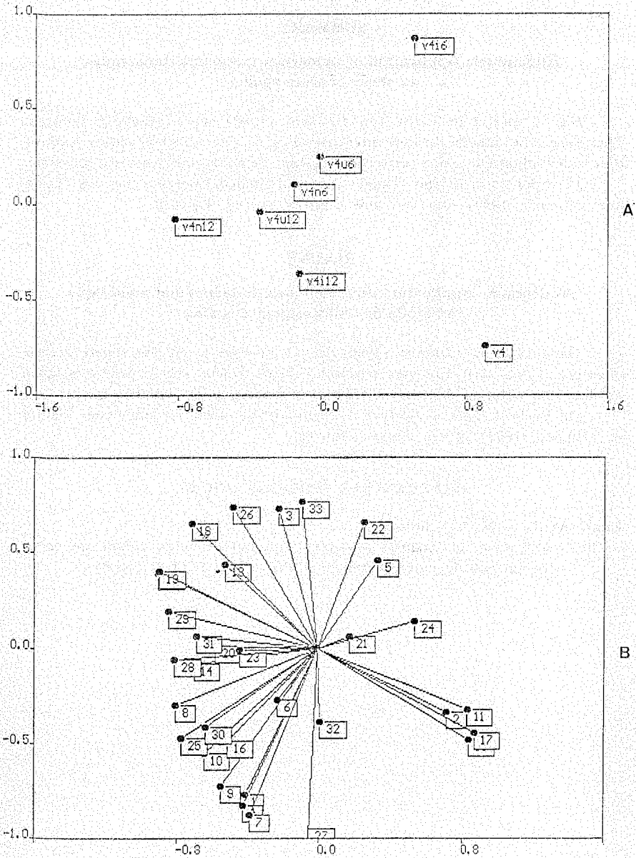
Fig. 2.2 — Projecções dos 7 vinhos da colheita de 1984 (A) e das 33 características (B) nos planos definidos pelos eixos principais I e II. Ver Anexo I para códigos de identificação.
