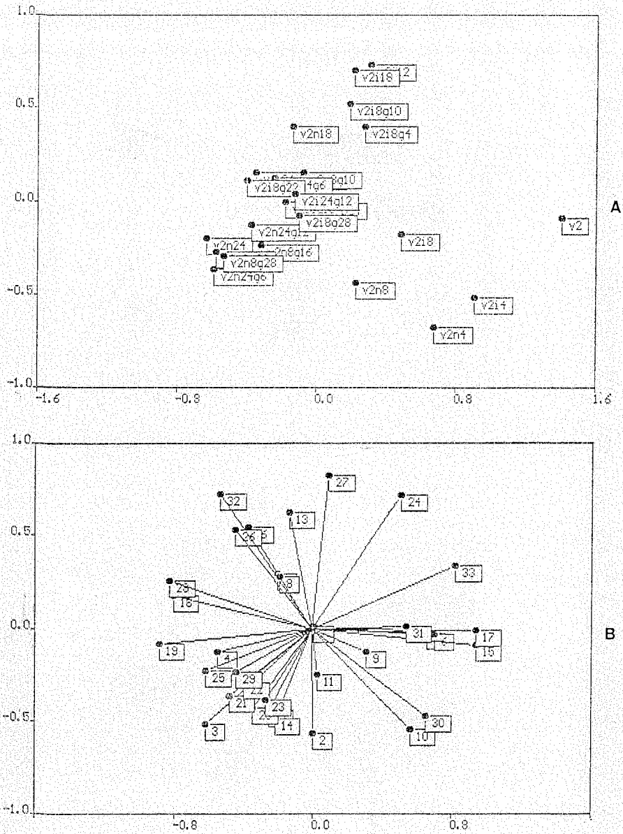
Fig. 1.2 — Projecções dos 25 vinhos da colheita de 1982 (A) e das 33 características (B) nos planos definidos pelos eixos principais I e II. Ver Anexo I para códigos de identificação.
