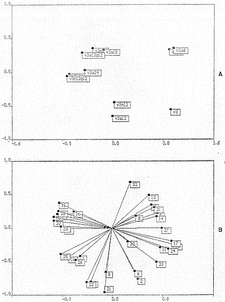
Fig. 2.1 — Projecções dos 11 vinhos da colheita de 1983 (A) e das 33 características (B) nos planos definidos pelos eixos principais I e II. Ver Anexo I para códigos de identificação.
