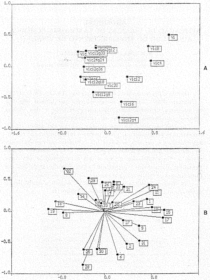
Fig. 1.1 — Projecções dos 18 vinhos da colheita de 1981 (A) e das 33 características (B) nos planos definidos pelos eixos principais I e II. Ver Anexo I para códigos de identificação.
