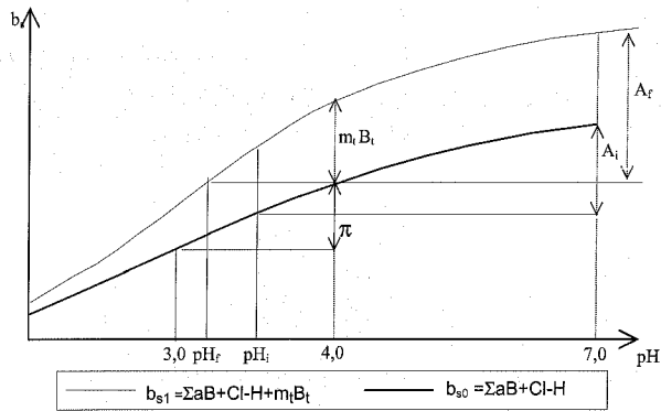
Fig. 1 - A adição de m_j mM/l de ácido tartárico. As duas curvas diferem m_j B_j mE do ácido utilizado.
